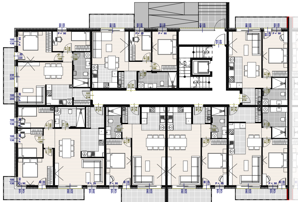
TLOCRT PRIZEMLJA
