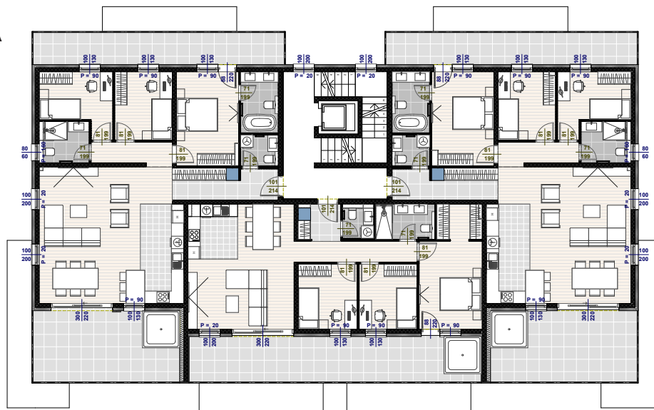
TLOCRT UVUČENOG KATA
