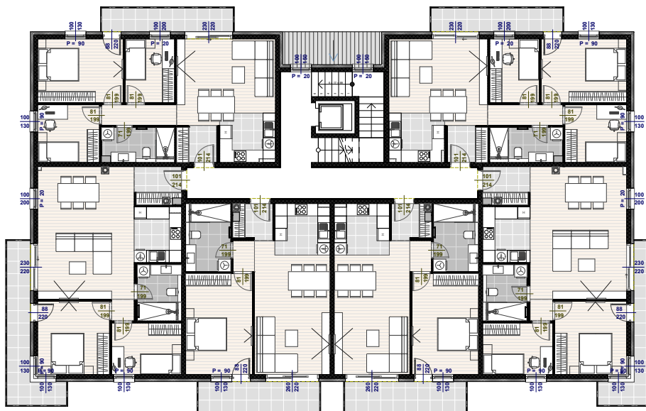
TLOCRT 1.KATA
